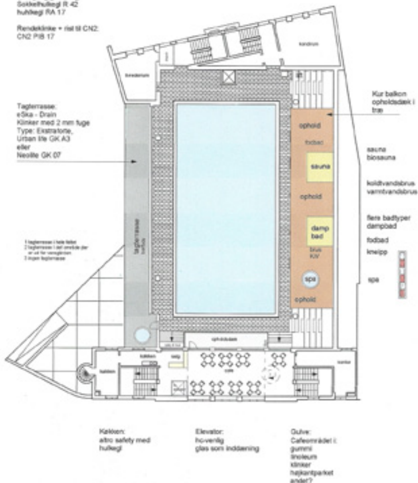
Plan over hal med terrasse (bade)
